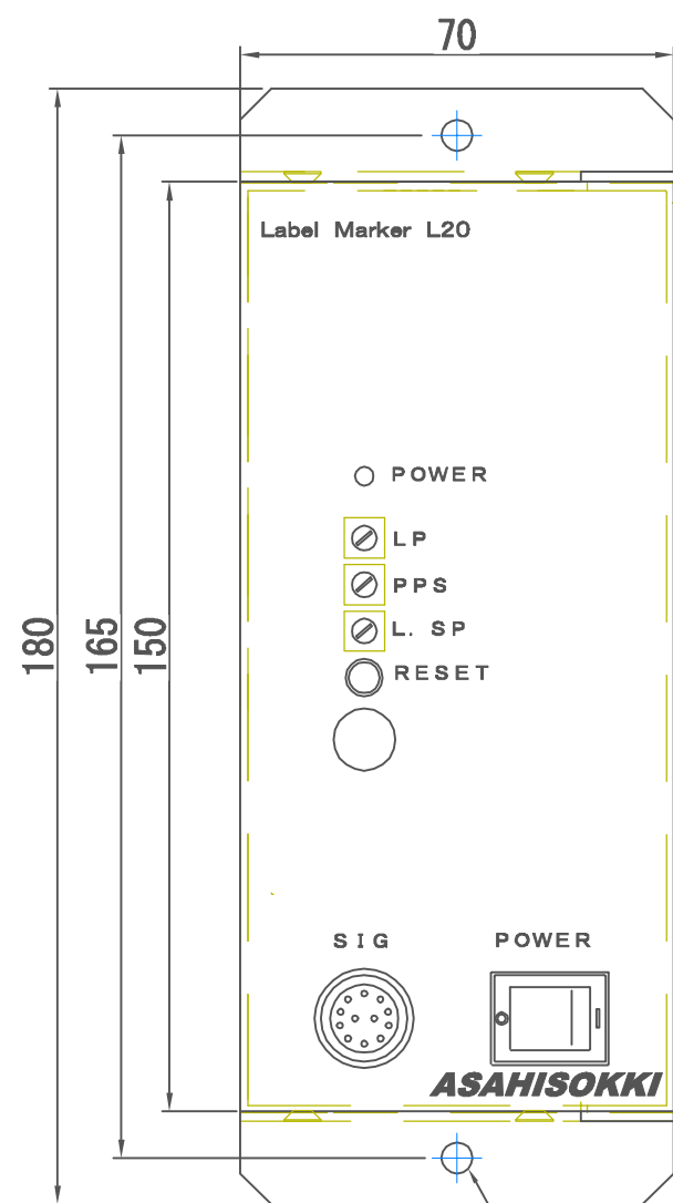
正面図 (Front view)
