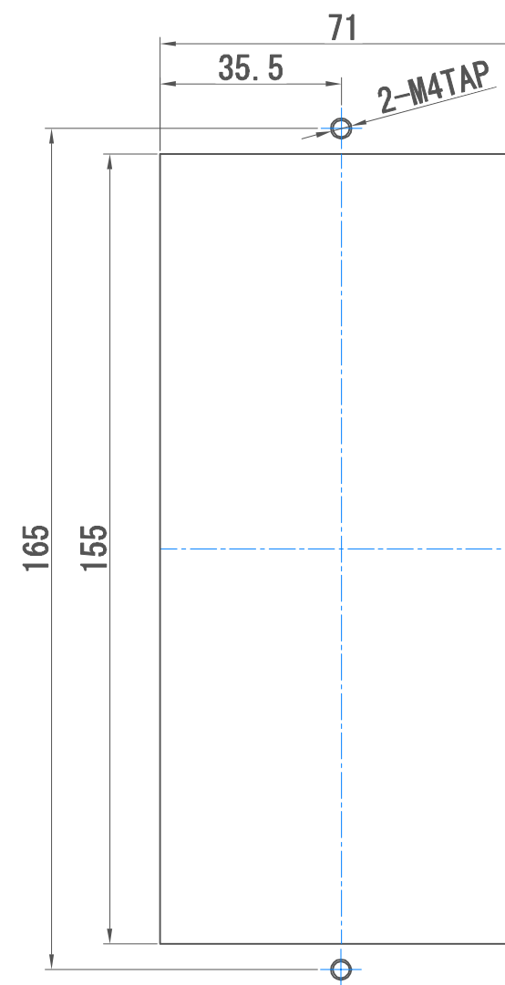
穴開け寸法図 Drilling dimension diagram
